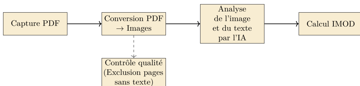
FIGURE 14 – Pipeline séquentiel de collecte, prétraitement et évaluation : de la capture web jusqu'au calcul de l'indice IMOD. — 7 septembre 2026
