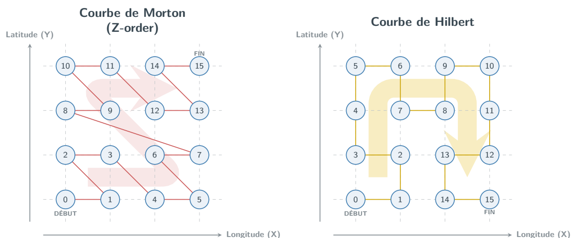
FIGURE G.3 – Comparaison des trajectoires des courbes de Morton (Z-order) et de Hilbert pour le parcours d'un espace matriciel bidimensionnel ( 4 \times 4 ). — 7 septembre 2026
