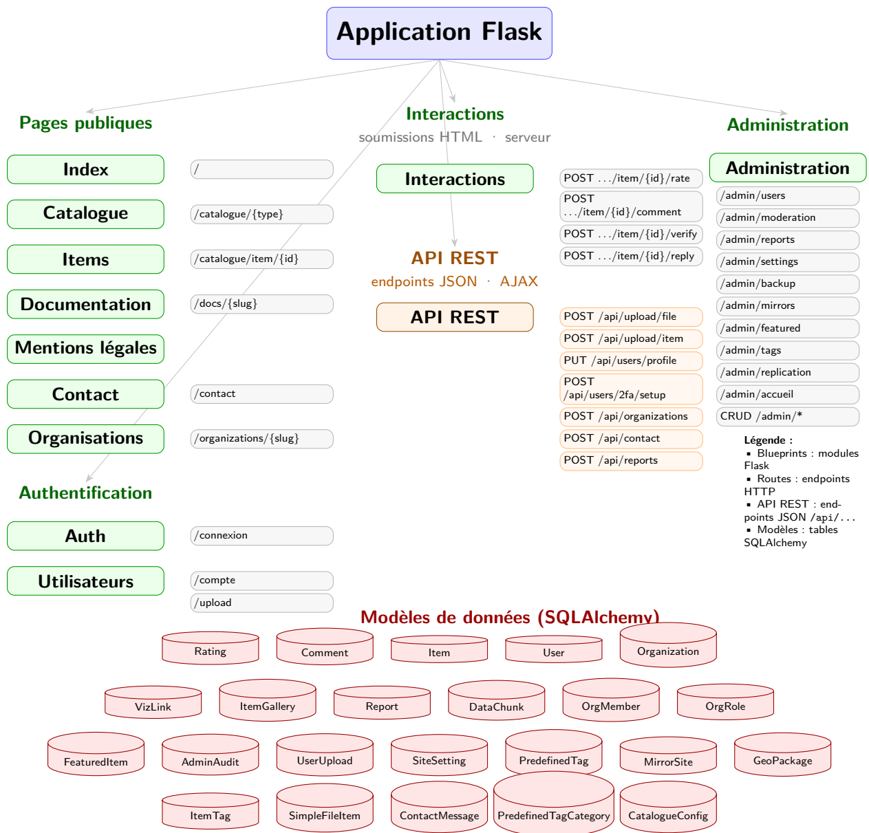
FIGURE F.2 – Architecture applicative – blueprints, routes et modèles. — 7 septembre 2026
