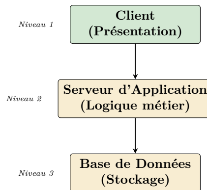
FIGURE 3 – Schéma d'une architecture client-serveur à trois niveaux (3-tier) illustrant la séparation des responsabilités. — 7 septembre 2026
