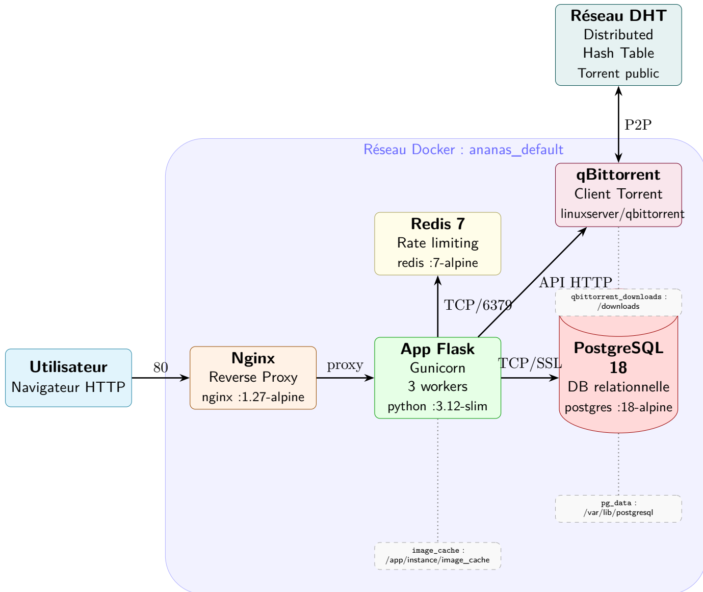
FIGURE F.1 – Architecture système – déploiement et services. — 7 septembre 2026
