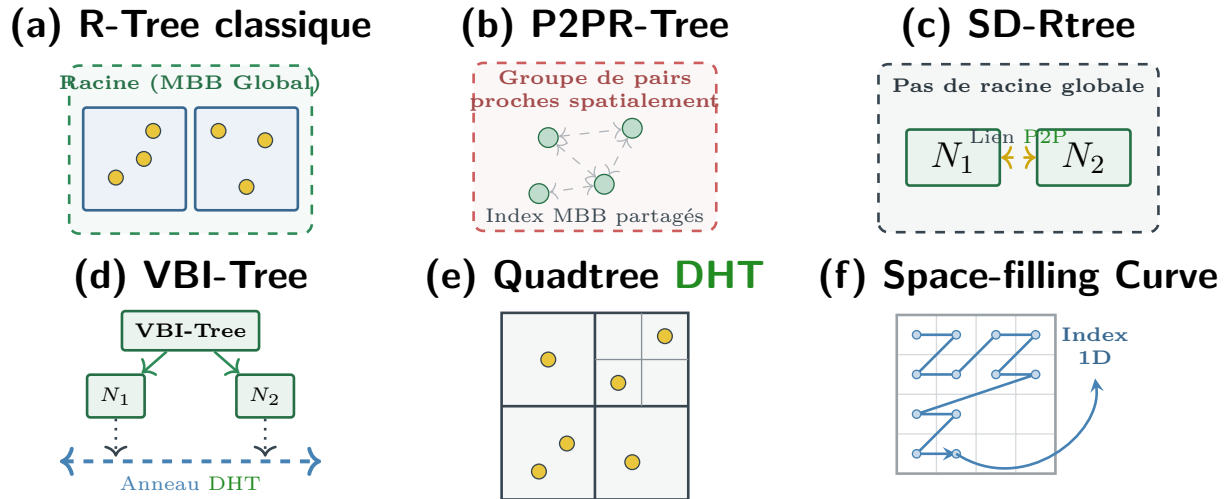
FIGURE 11 – Principes fondamentaux des structures d'indexation spatiale distribuée. — 7 septembre 2026
